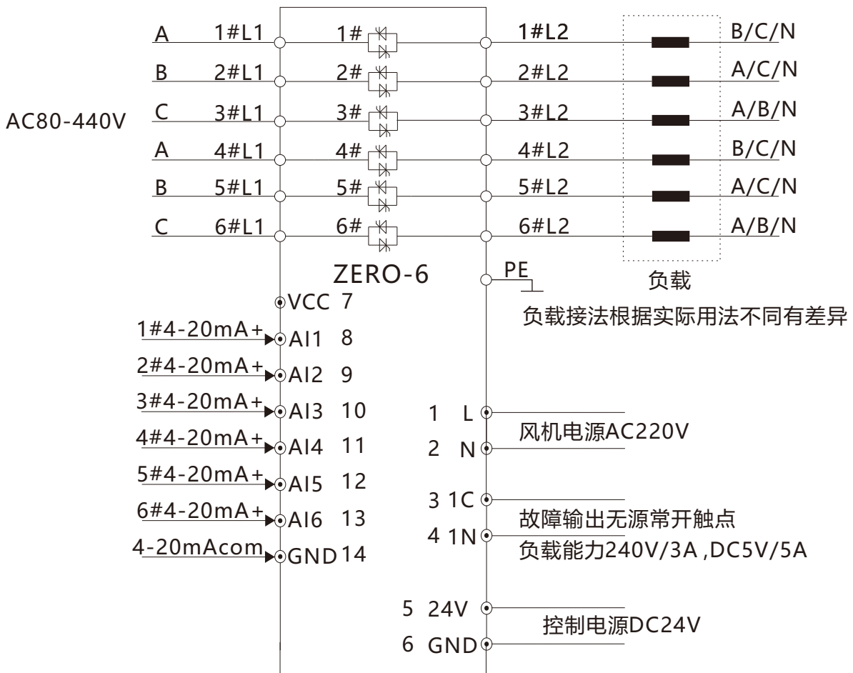
主回路、控制回路配线图
